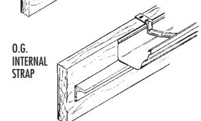
HI-TEN O.G. GUTTER
